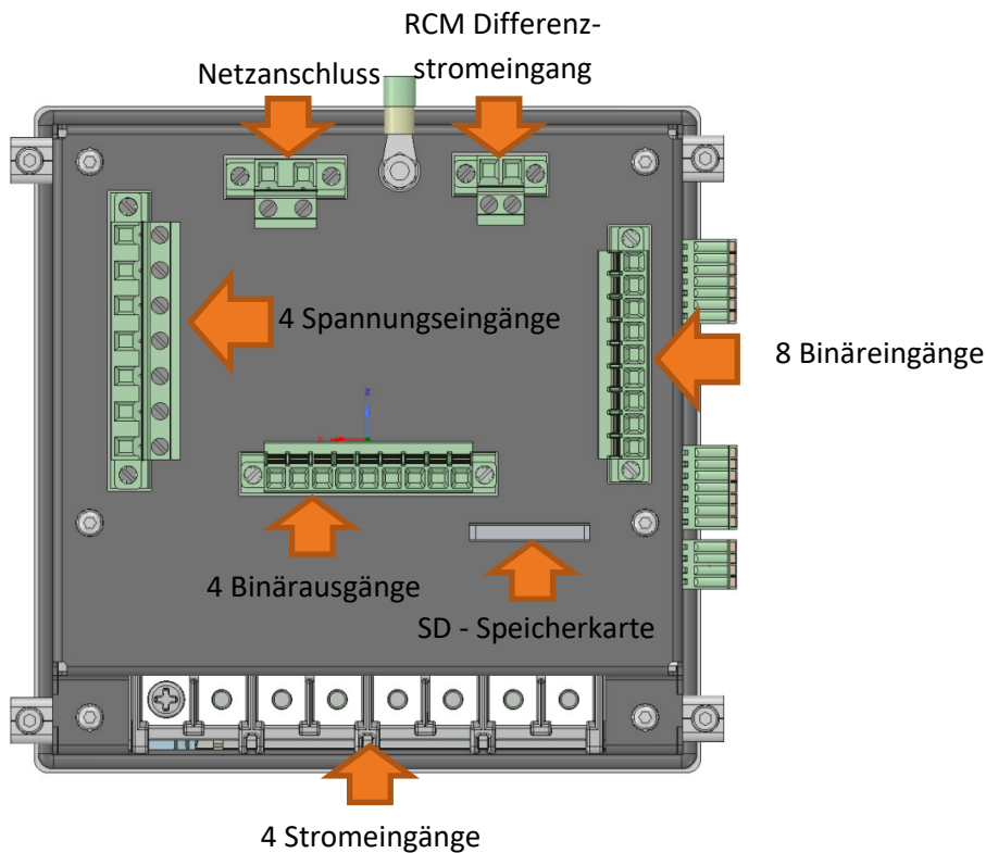
Rückansicht PQI-DE
